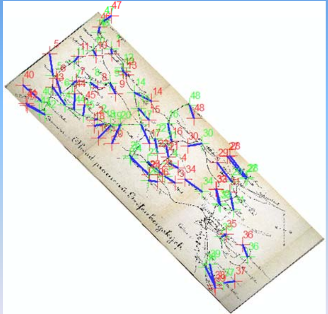
Vektory posunů při afinní transformaci Obvod pramenů Gréfenbergských [1] [autorka]
